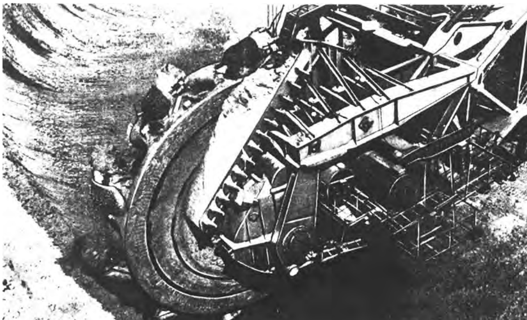
Роторный экскаватор комплекса «Михайловка-2» вгрызается в толщу горных пород
