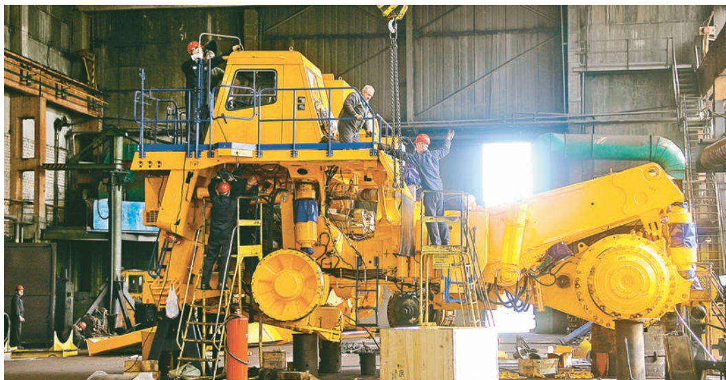
В боксе УАТ идет монтаж большегруза
